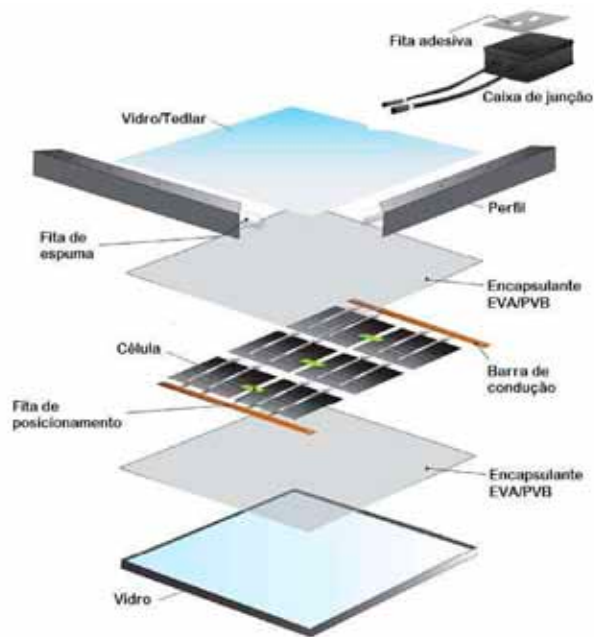
Fig. 5.9 Componentes de um módulo fotovoltaico de silício cristalino. Adaptado de Homero Schneider, Inova FV (2011). Há módulos de filmes finos sem molduras, em sanduíche vidro-vidro.
