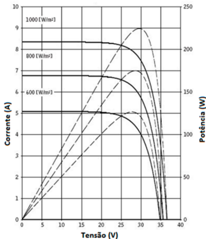
Fig. 5.8 – Curva característica de módulo fotovoltaico.
