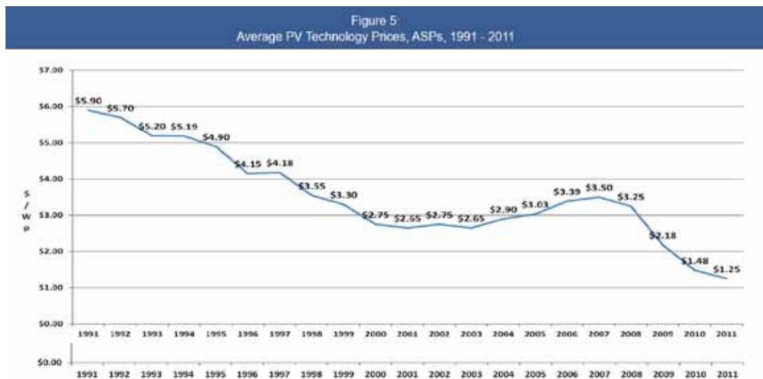
Fig. 5.25 – Preço médio dos módulos fotovoltaicos. Fonte: Navigant's Solar Outlook 2012-01 (Fev 2012).
