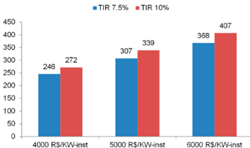
Fig. 2.14 – Preço de venda de contratos de 25 anos (R$/MWh) com incentivos fiscais análogos aos oferecidos aos projetos de energia eólica. Amortização SAC.
