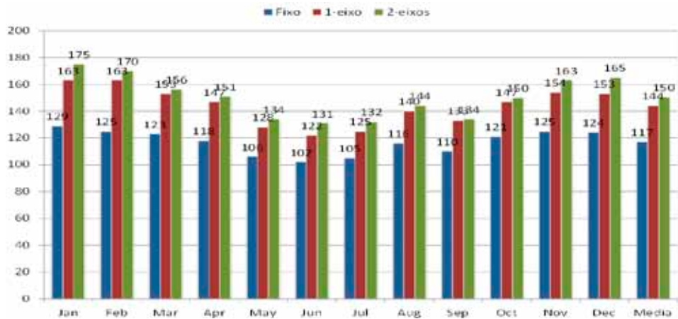
Fig. 5.23 – Acima: sistema fixo, com rastreamento de um e dois eixos. Abaixo: correspondente produção de energia fotovoltaica (Wh) para instalação de 1000 Wp no RJ. Há ganho de +23% e 28% na produção anual de energia para rastreadores com rotação de 1 e 2 eixos, respectivamente.
