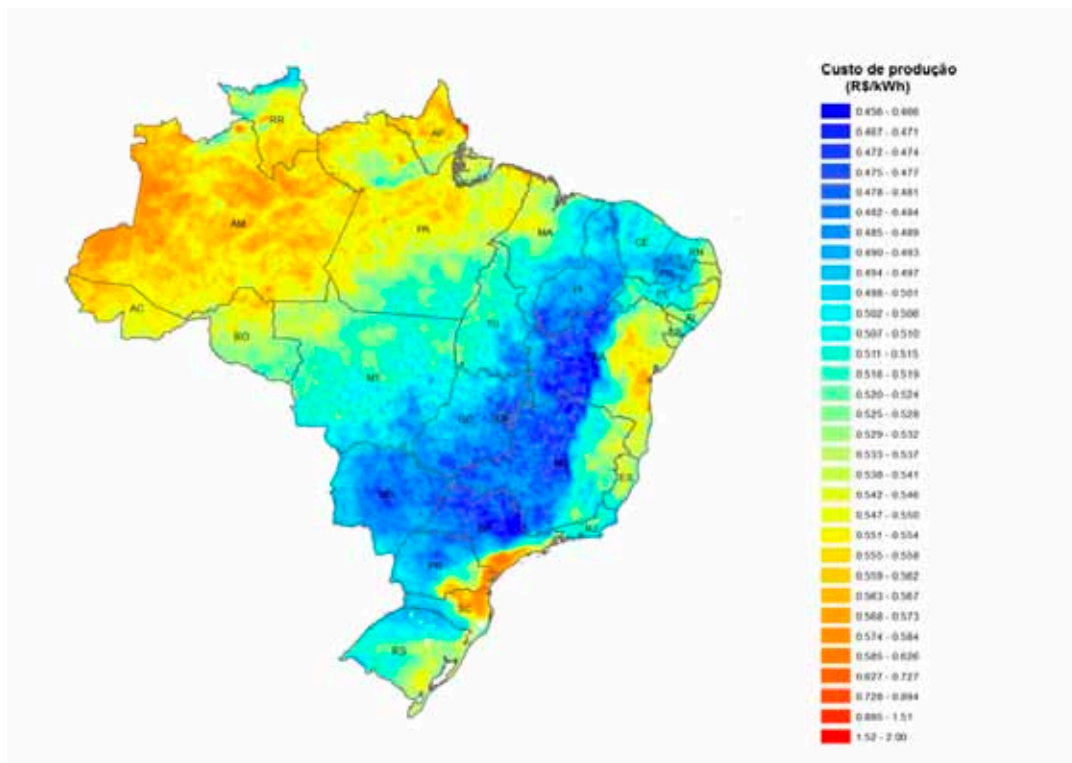
Fig. 2.6 – Custo de produção de energia (R$/kWh). Quanto mais fria a cor, menor o custo. Observam-se regiões propícias na faixa mais central do país cobrindo oeste dos Estados de SP, MG e BA; todo o PI, leste de TO, MA, e GO, além de faixa no sertão do CE, PB, RN, e RN.
