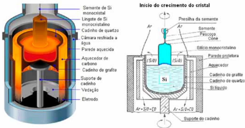
Fig. 5.15 Esquema de solidificação pelo método Czochralski para obtenção do lingote monocristalino. (Fonte: http://people.seas.harvard.edu .)
