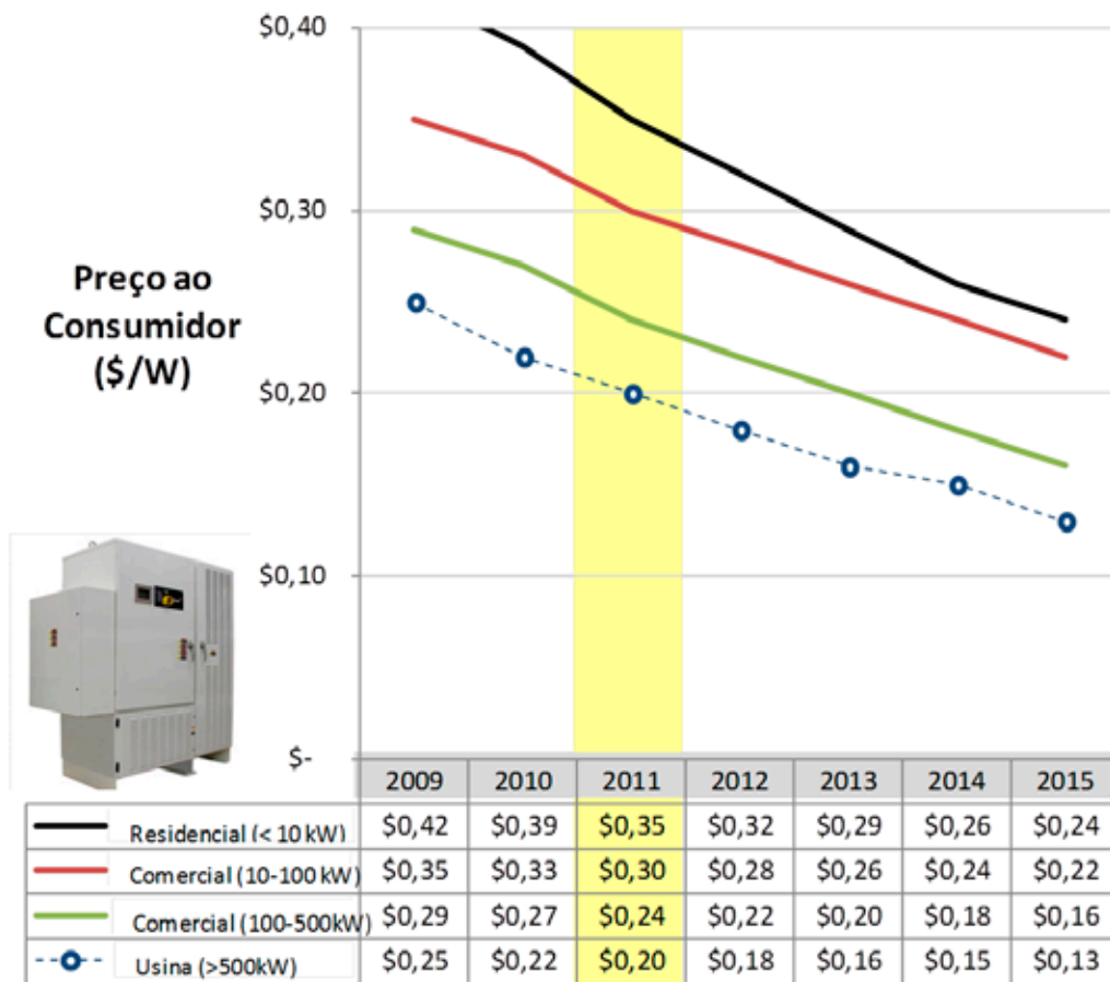
Fig. 6.8 Preços de inversores. (Fonte: GTM Research, jun/11)
