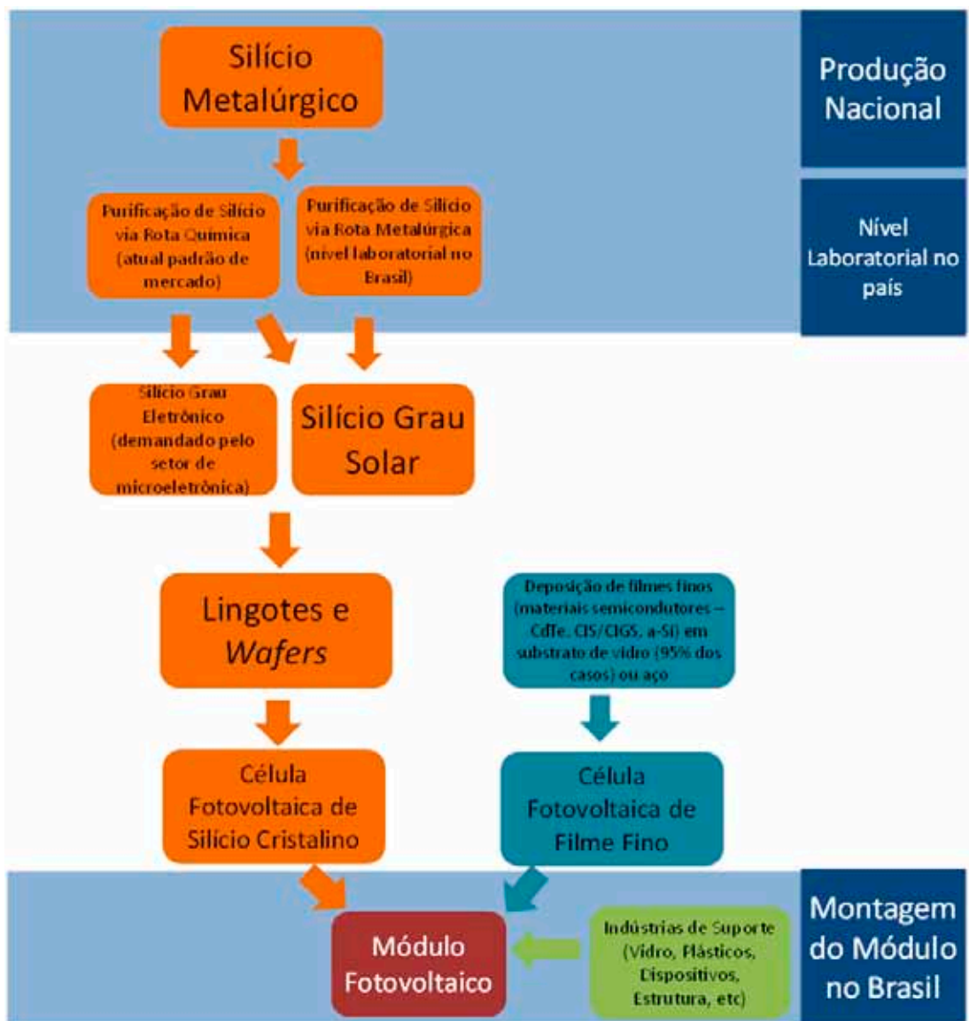
Fig. 1.3 – Cadeia de produção do módulo fotovoltaico.
