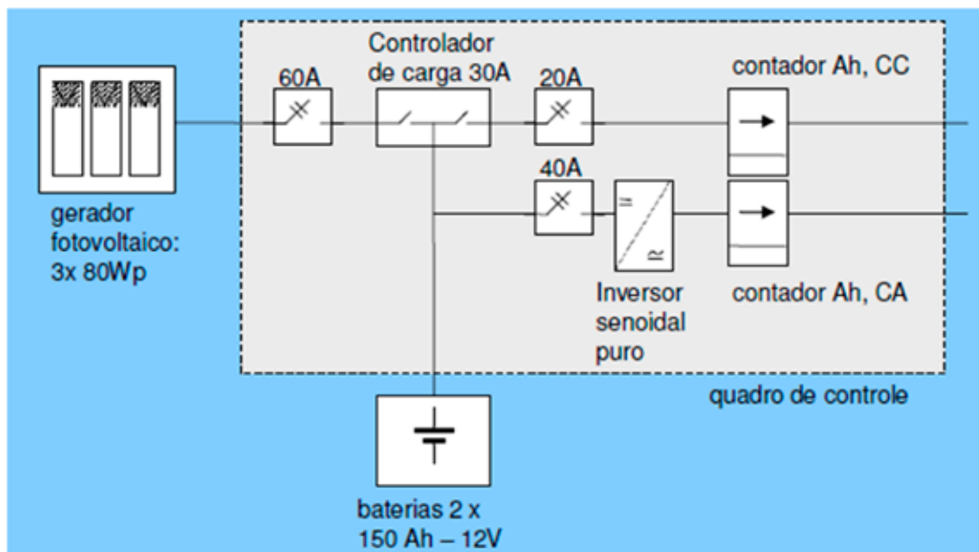
Fig. 1.2 – Sistema híbrido de 240 Wp. Fonte: Programa Luz para Todos, Eletrobras.
