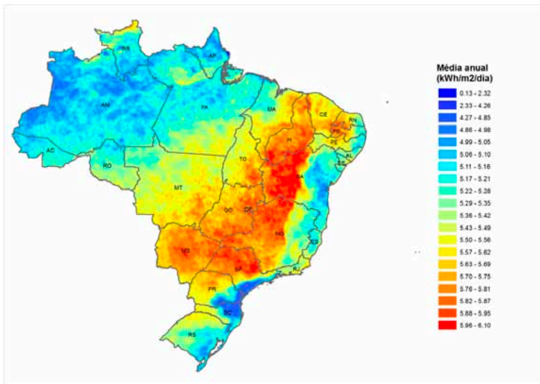
Fig. 2.1 – Irradiação total em plano cuja inclinação é igual a latitude do local. Mapa elaborado pela PSR com dados do projeto SWERA. Fonte: brazil_solar_tilted_10km.shp . O arquivo “shapefile” apresenta os dados de radiação solar em kWh/m 2 /dia para células 10km x 10km.
