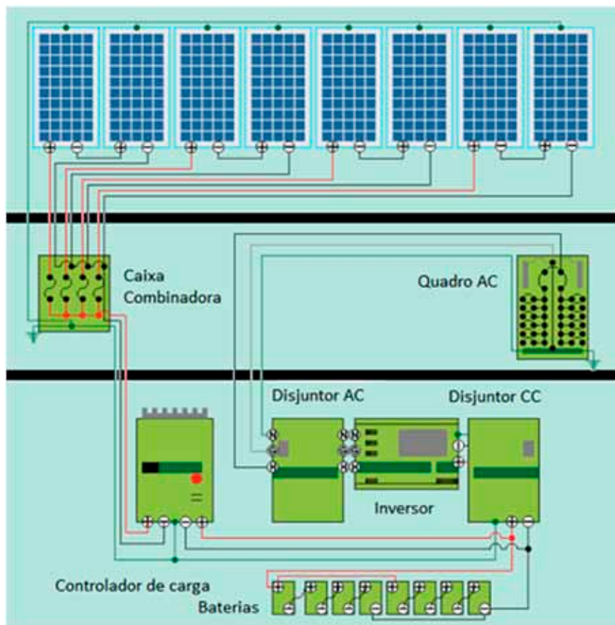
Fig. 5.7– Componentes de um sistema fotovoltaico isolado.
