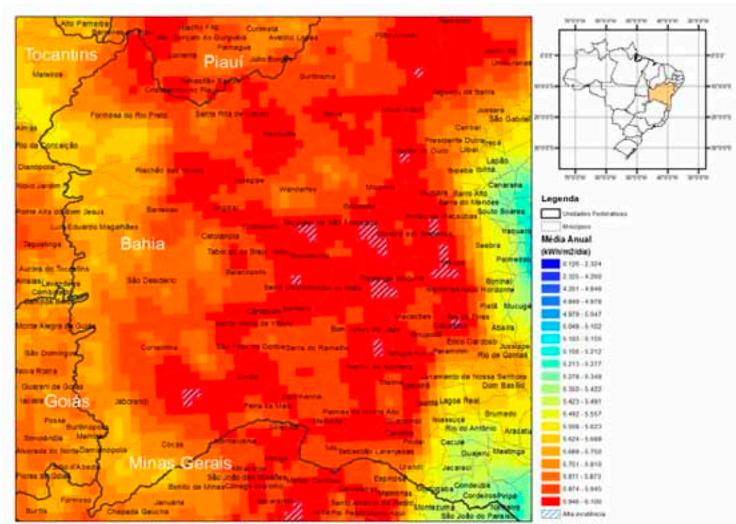
Fig. 2.13 – Hachuras do mapa indicam regiões com alta irradiação.
