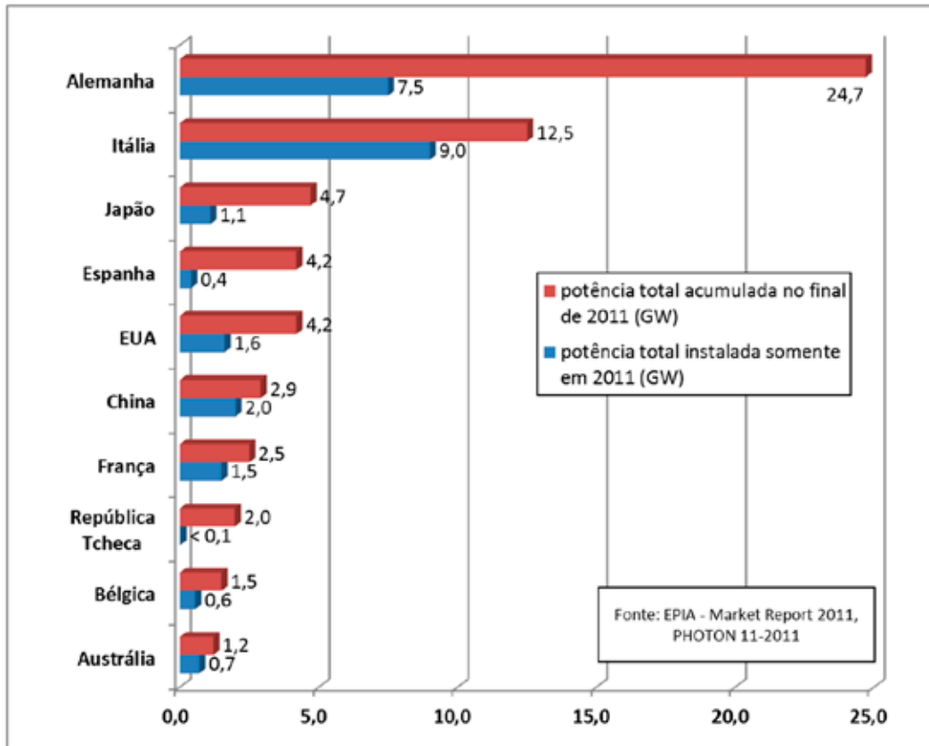
Fig. 5.26 – Principais mercados mundiais em 2010 (em GWp instalados). Fonte: EPIA – Market Report 2011, PHOTON Internacional 11-2011.
