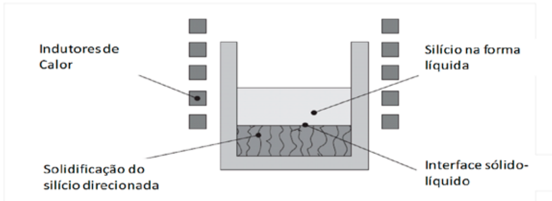
Fig. 5.14 Técnica de Bridgman para fabricação de lingotes de silício policristalino. (Fonte: Handbook of Photovoltaic Science and Engineering, 2nd Ed, 2011)
