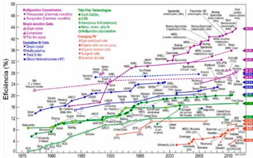
Fig. 7.8 Eficiência de conversão das células FV. Fonte: National Renewable Energy Lab (NREL).
