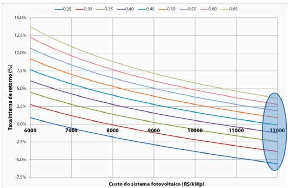
Fig. 1.7 – Taxa interna de retorno (TIR) real (sem inflação) de sistema fotovoltaico em função do custo de instalação e tarifa final da concessionária com impostos (variando entre 0,25 R$/kWh e 0,65 R$/kWh).
