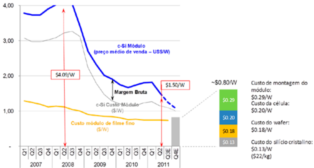
Fig. 6.5 Custo e preços dos módulos, considerando a distribuição de custos do módulo de silício cristalino de menor custo. (Fonte: YingLi, Trina Solar, First Solar, Solar Buzz, Deutsche Bank.)
