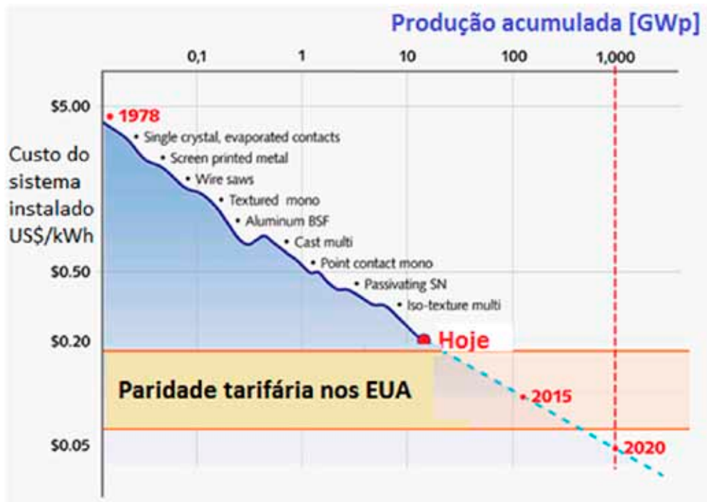
Fig. 5.29 – Evolução de preço da energia fotovoltaica (US$/kWh) em função do total produzido acumuladamente. Gráfico adaptado do Prof. Emanuel Sachs, MIT. No curto prazo (<10 anos) a energia fotovoltaica supera a paridade com formas convencionais de energia baseadas em combustíveis fósseis. O limite superior da banda de paridade representa o custo de produção de térmicas a gás natural para atendimento da demanda de ponta, enquanto que o limite inferior representa o custo de produção de usinas térmicas a carvão que despacham “na base”.
