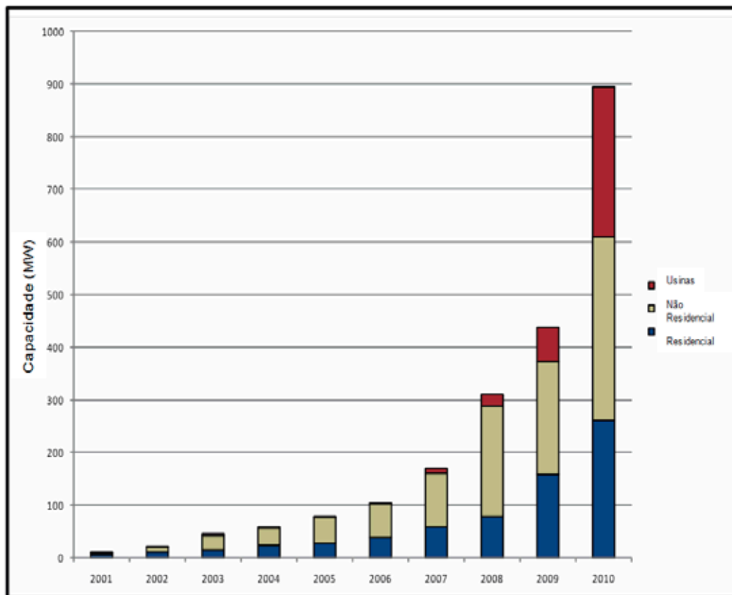
Fig. 3.4 – Potência instalada em geração fotovoltaica, por setor (Fonte: IREC Report 2011).
