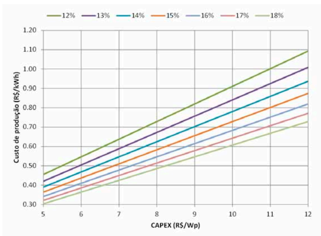
Fig. 2.5 – Custo de produção de energia (R$/kWh) para faixas de custo instalação (eixo X) e “famílias” de curvas com fatores de capacidade variando entre 12% e 18% (legenda na parte superior do gráfico).
