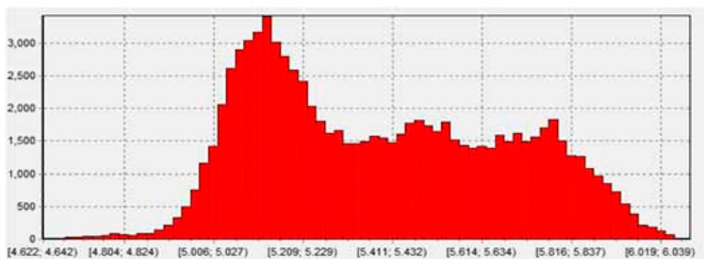
Fig. 5.4 – Histograma com irradiação em plano inclinado igual à latitude do local. Observa-se grande ocorrência de irradiação em nível superior a 4,8 kWh/m 2 /dia. Fonte: SWERA.
