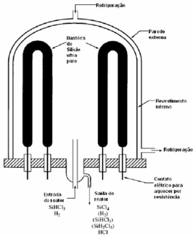
Fig. 5.12 Desenho esquemático do Reator Siemens. (Fonte: RIMA Industrial)
