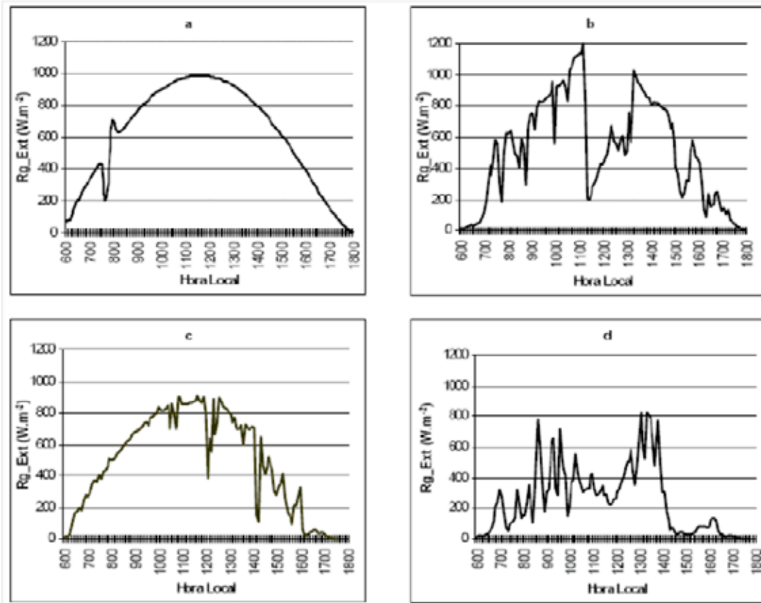
Fig. 2.2 – Radiação Solar Global ( W/m^2 ), a cada cinco minutos, na ilha de Santa Rita, município de Marechal Deodoro – AL (QUERINO, C. A. S. et al. “Estudo da Radiação Solar Global e do Índice de Transmissividade (KT), Externo e Interno, em uma Floresta de Mangue em Alagoas – Brasil”. Revista Brasileira de Meteorologia, v. 26, n. 2, 204-294, 2011). (a) 17 de janeiro, (b) 09 de fevereiro, (c) 01 de junho e (d) 31 de maio de 2005.
