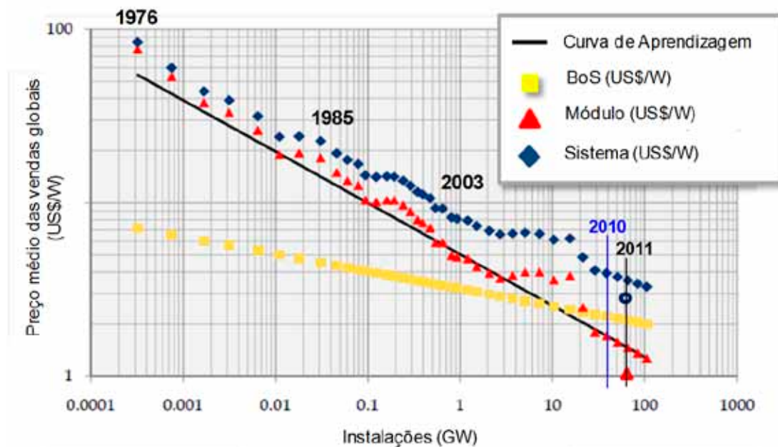
Fig. 6.10 Curva de aprendizagem do setor fotovoltaico. Preços ao consumidor x potência instalada. (Fonte: DoE, 2010.)
