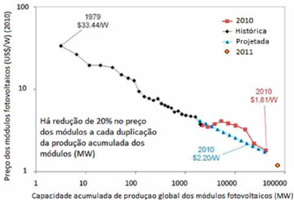
Fig. 2.16 – Curva de aprendizado tecnológico para módulos fotovoltaicos
