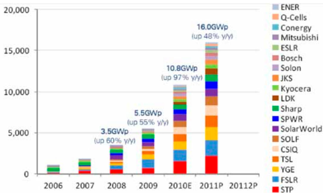
Fig. 6.4 Embarques de módulos solares, em MWp/ano. Os cinco principais players listados são Suntech Power (STP), First Solar (FSLR), Yingli Green Energy (YGE), Trina Solar (TSL) e Canadian Solar (CSIQ). (Fonte: Deutsche Bank.)
