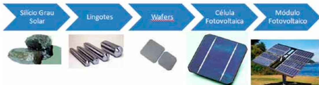
Fig. 5.17 Cadeia produtiva do módulo fotovoltaico baseado em silício cristalino. (Imagens: IPT, CEEG, Inovação Tecnológica.)
