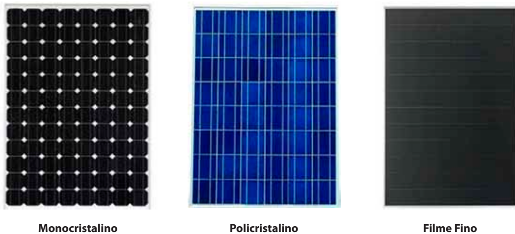
Fig. 5.11– Módulos fotovoltaicos mais comuns. O corte nas células de silício monocristalino tem formato circular, porém, o ideal é que ocupem a maior área possível. Por isso pequenos cortes são feitos, de modo que a célula redonda se assemelhe a um octógono (esq.). Ao centro, módulos policristalinos com tradicional aspecto azulado. A escassez relativa de silício no mercado entre 2005 e 2009 e o surgimento de empresas oferecendo linhas de produção turn key para células de filme fino (direita) provocaram rápida expansão nesta tecnologia, com o surgimento de cerca de 200 empresas.
