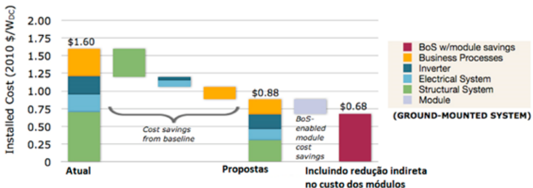
Fig. 2.18 – Redução no custo do chamado “BOS”, que incluem todos componentes (inclusive serviços) com exceção dos módulos. Fonte: Rocky Mountain Institute.
