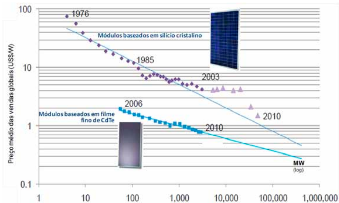
Fig. 6.6 Preços dos módulos. Ajustes de inflação foram feitos utilizando o PPI americano. O R2 das curvas estimadas foi de 0,94 para módulos de silício cristalino e 0,98 para módulos de CdTe. (Fonte: Bloomberg New Energy Finance)
