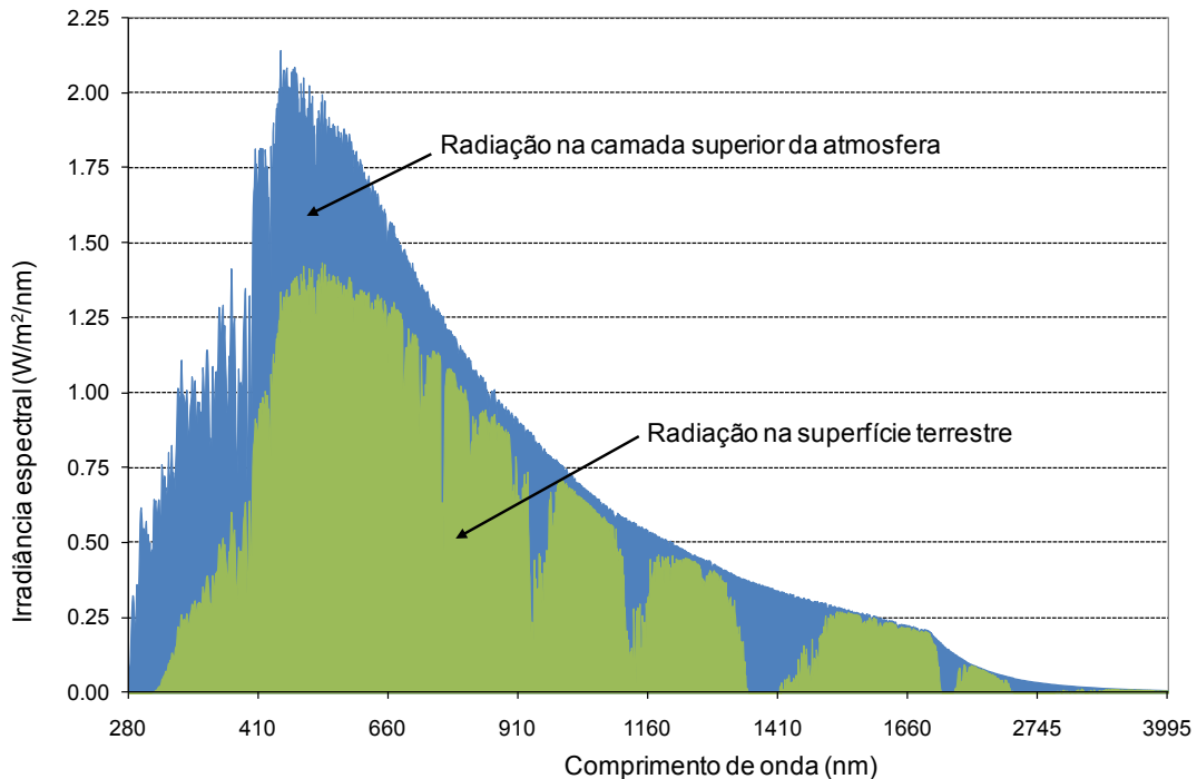
Fig. 5.1 – Radiação espectral (fonte: NASA)
