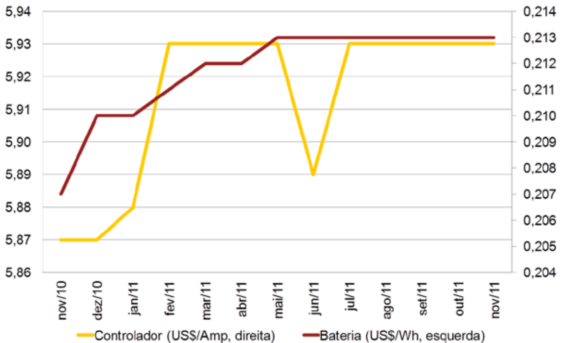
Fig. 6.9 Preço médio de baterias e controladores de carga. (Fonte: Solarbuzz, 2011.)
