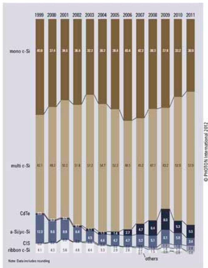
Fig. 5.10– Participação das células fotovoltaicas na produção total.
