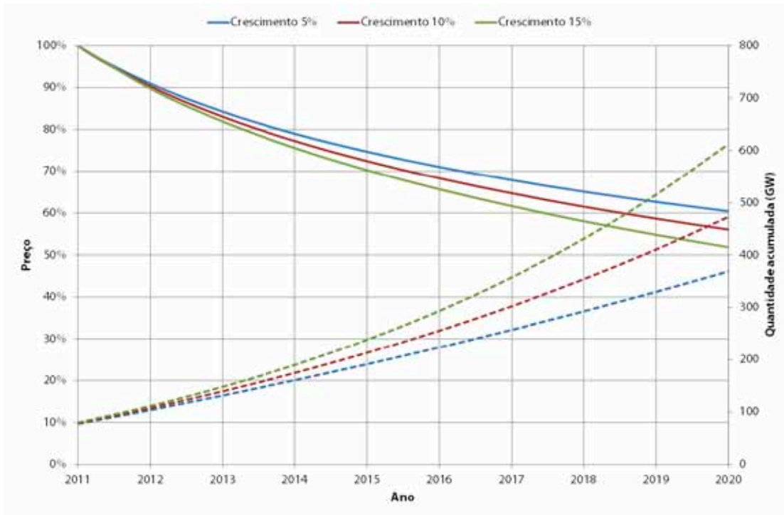
Fig. 2.17 – Curva de aprendizado tecnológico para módulos fotovoltaicos
