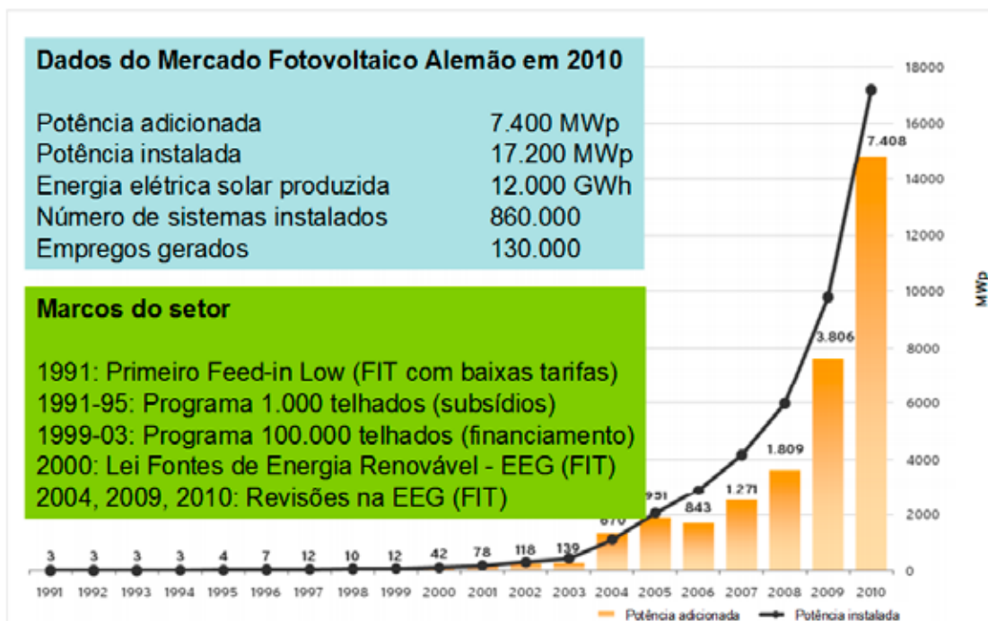
Fig. 3.2 – Dados do mercado fotovoltaico alemão em 2010. (Fonte: BSW Solar / www.solarwirtschaft.de ).
