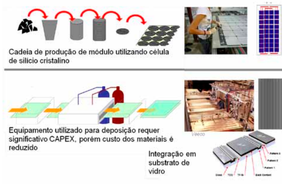
Fig. 5.19 Diferenças nos processo de fabricação de módulos utilizando silício cristalino (na parte superior) e filme fino, com deposição em substrato de vidro (parte inferior). Os custos relacionados ao material utilizado na produção de células com silício cristalino têm absorvido boa parte dos recursos de P&D no setor ao longo dos anos. (Fonte: Saint-Gobain Solar)
